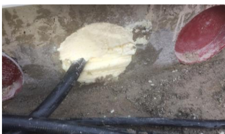
Rohreingang mit COVERSOL® versiegelt
